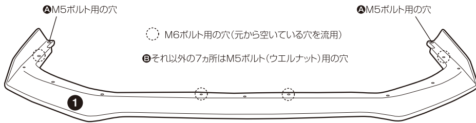
*穴あけ後右図を参考に、7カ所に付属のウエルナットの取付け作業を行ってください。
