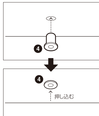
次に付属のウエルナットを穴にセットします。
