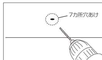
ドリル等を使用し7カ所の印位置に9mmの穴を開けてください。
