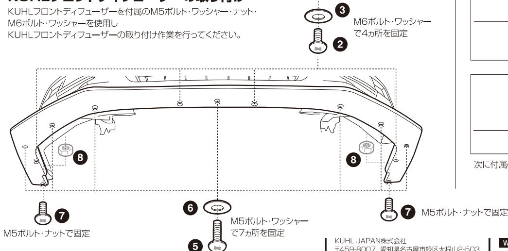
*穴あけ後右図を参考に、7カ所に付属のウエルナットの取付け作業を行ってください。
